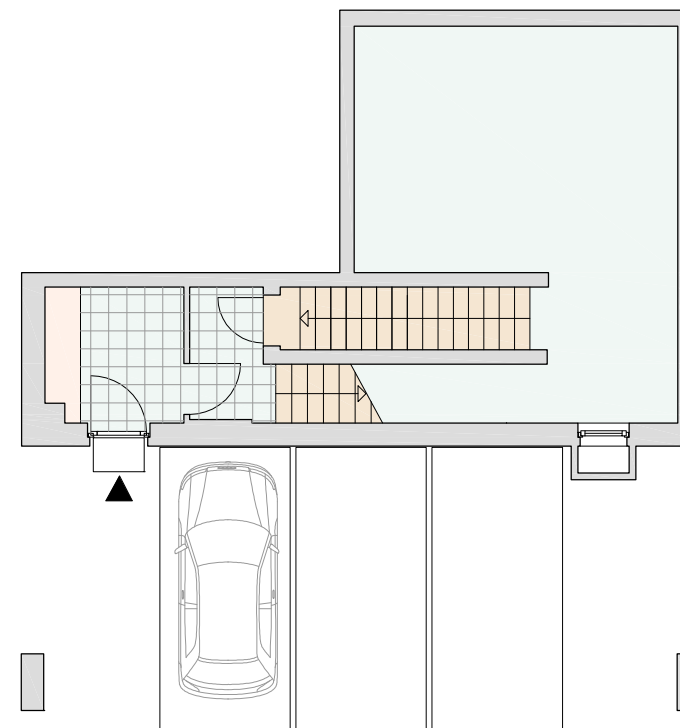
Erdgeschoss / Keller
